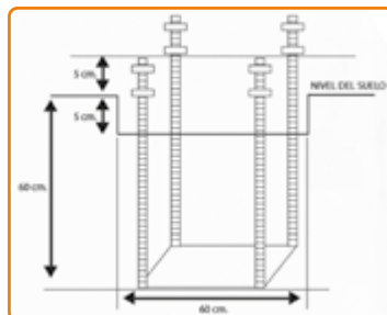
Detalle del hormigonado de anclaje para canasta fija. El anclaje se suministra con la canasta.
